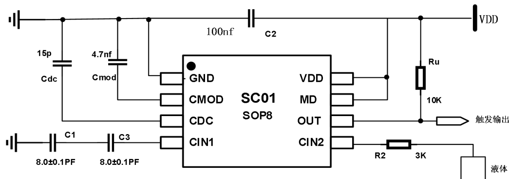
图 3-1：水位检测或者人体检测应用电路
