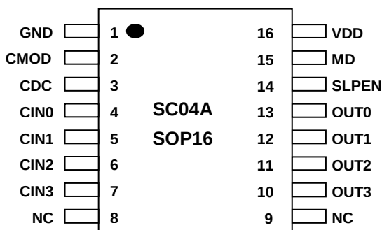
图 1-1: 封装简图
