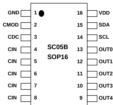
图 1-1: 封装简图
