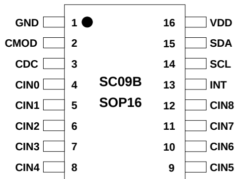
图1-1: 封装简图
