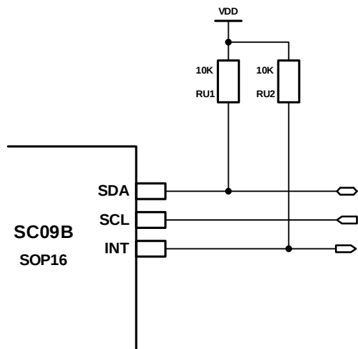
图3-2: I 2 C 中断方式
