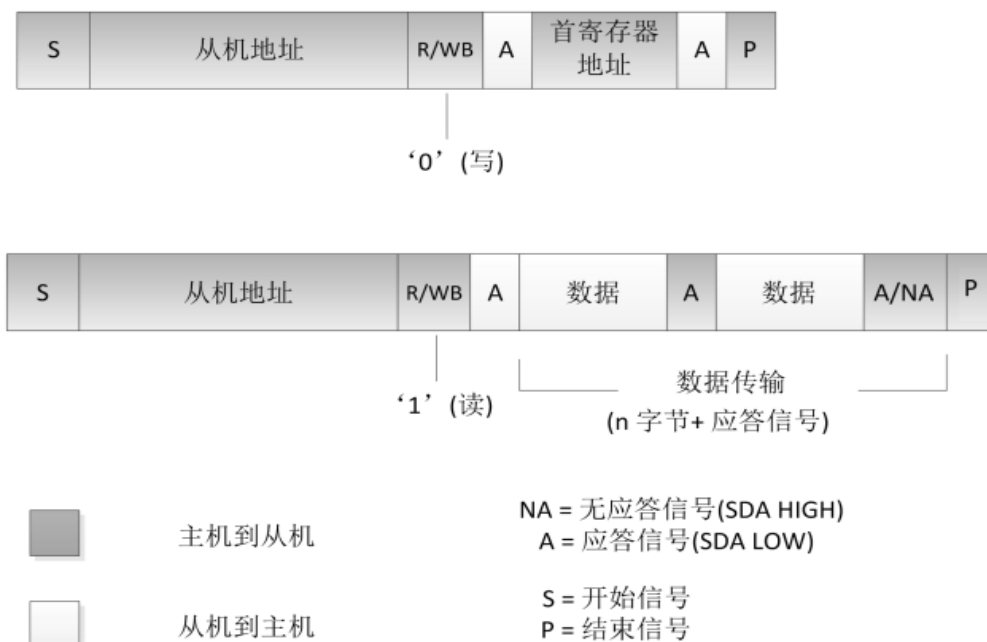
图 3-7 : 读操作
