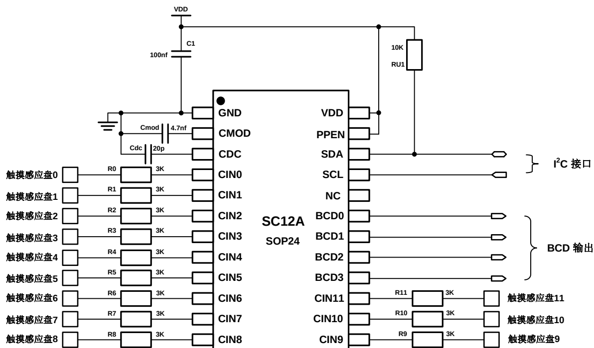
图 3-1 : 应用电路
